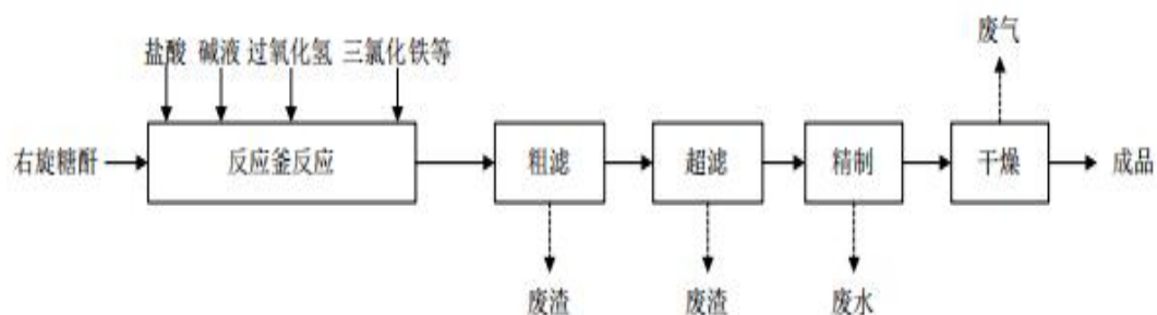
图 3.1.3-1 原料药车间生产工艺流程
